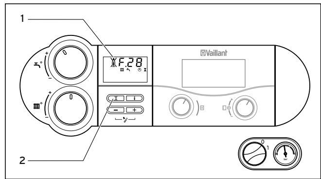
Abb. 4.13 Entstörung
