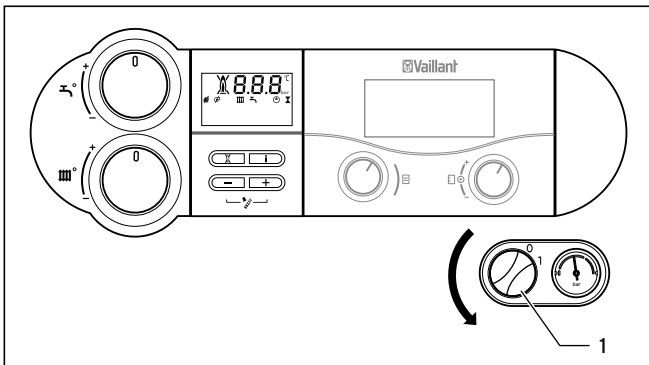
Abb. 4.15 Gerät ausschalten
